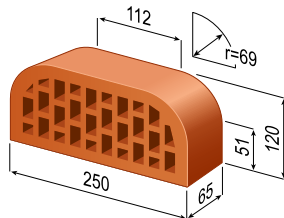
Цегла з двома закругленими краями
