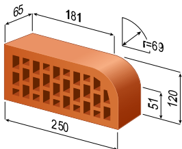
Цегла з одним закругленим краєм
