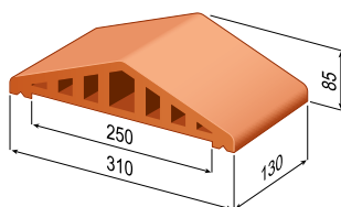
Навіс на стіну DD
