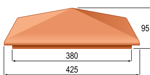
Ковпак на стовпчик
